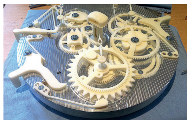
Maquette d'une planche additionnelle: quantième annuel spécial avec module Lune de précision
