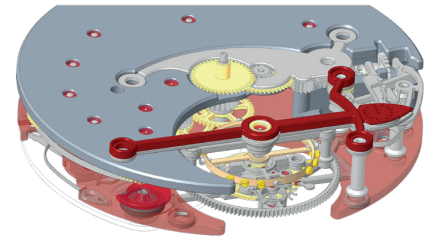
Visuel 3D: tourbillon avec stop seconde à blocage indexable invisible, et masse à rotation limitée
